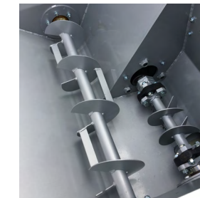
Zusätzliche Rührwelle im 400 Liter Förderbehälter
